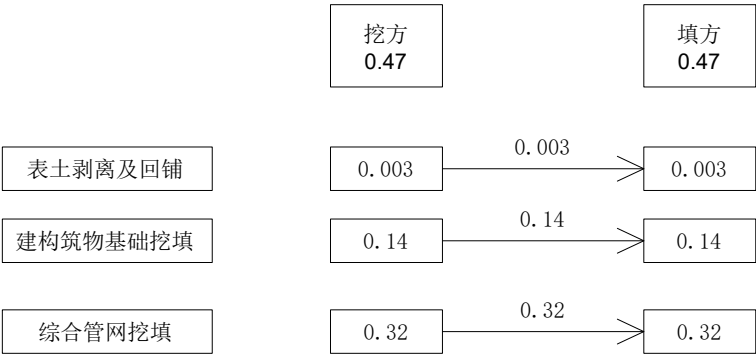
图 2.4-1 土石方平衡流向框图
