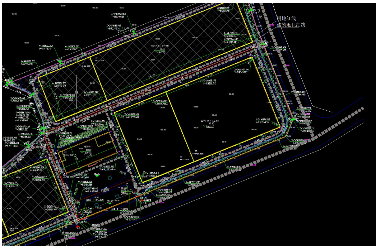
图 2.1-3 项目总平面布置图
